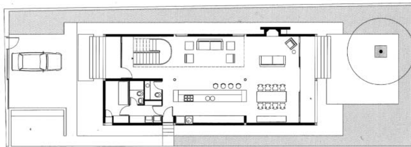
Residência no Butantã, São Paulo, SP, 2004 Plantas
