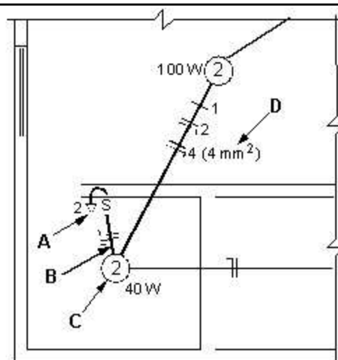
Hélio Creder. Instalações elétricas, p. 54 (com adaptações).
